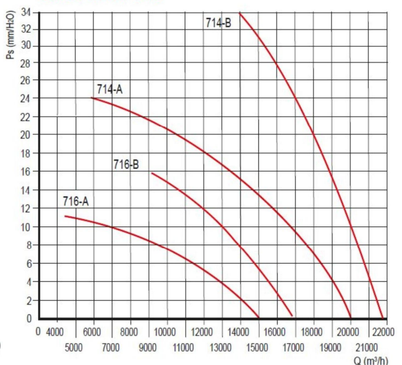
DUCT-M-HT 710
