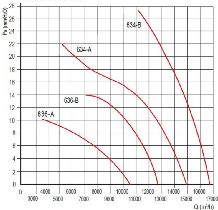
DUCT-M-HT 630
