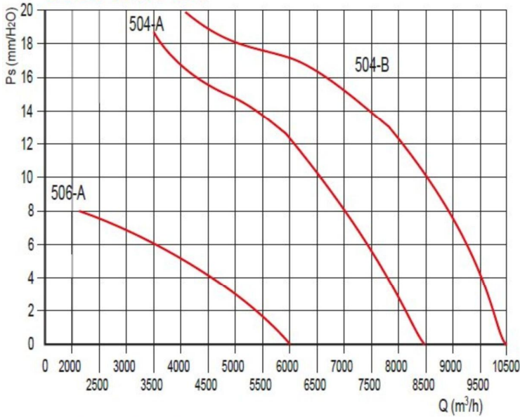
DUCT-M-HT 630
