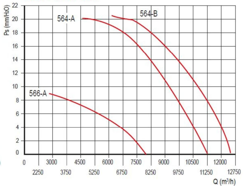
DUCT-M-HT 710
