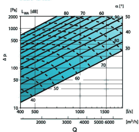
AKH Ø400
