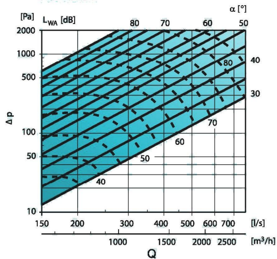
AKH Ø250
