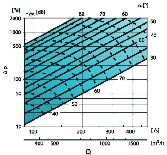
AKH Ø200
